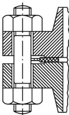
Joint à anneau de centrage
