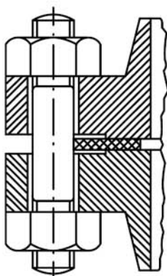
Joint à autocentrage
